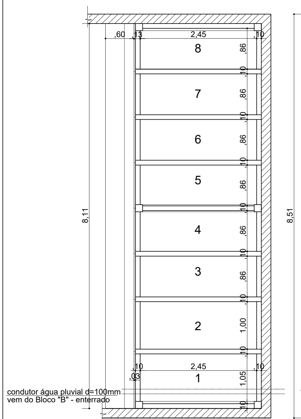
PLANTA BAIXA - BLOCO "A" ESC.: 1/50 A= 21,73m 2
