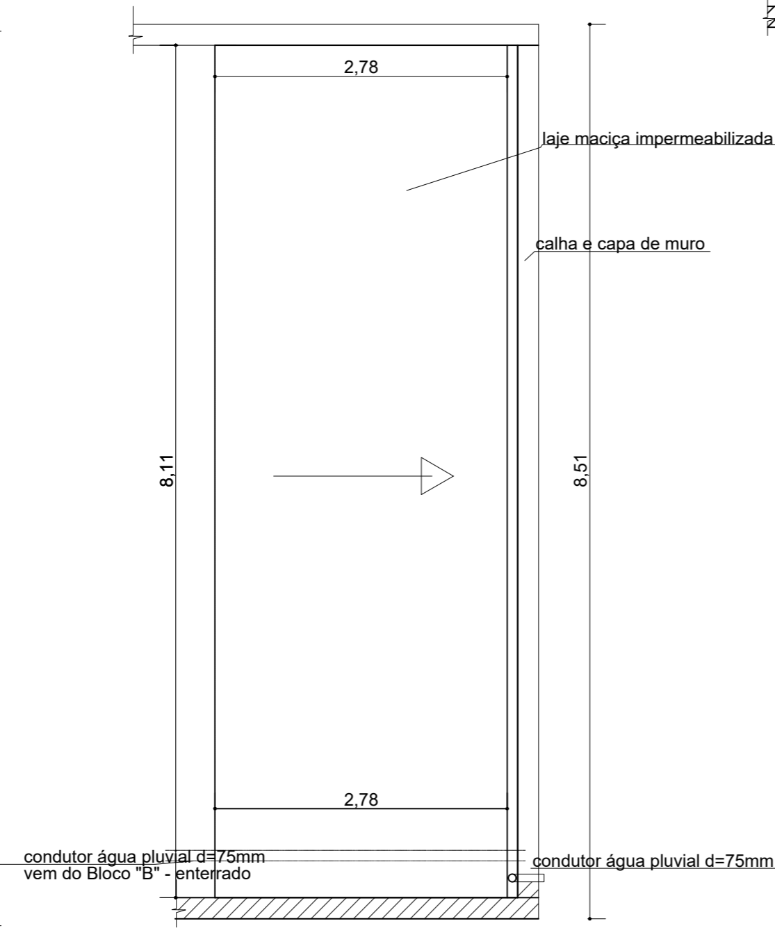
PLANTA DE COBERTURA - BLOCO "A"
