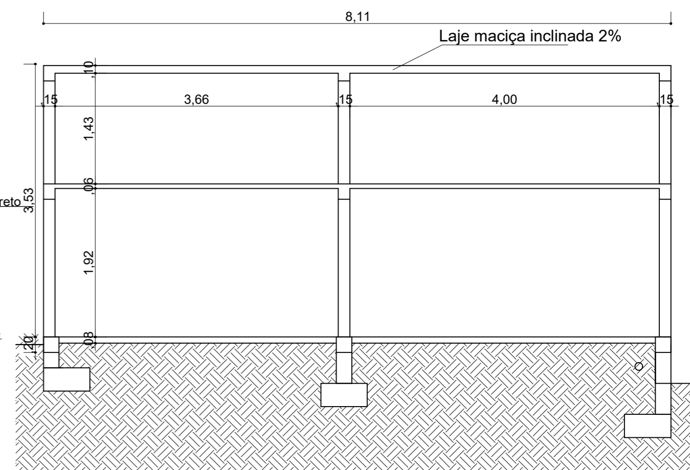
PROJETO ESTRUTURAL BLOCO "A" ESC.: 1/50
