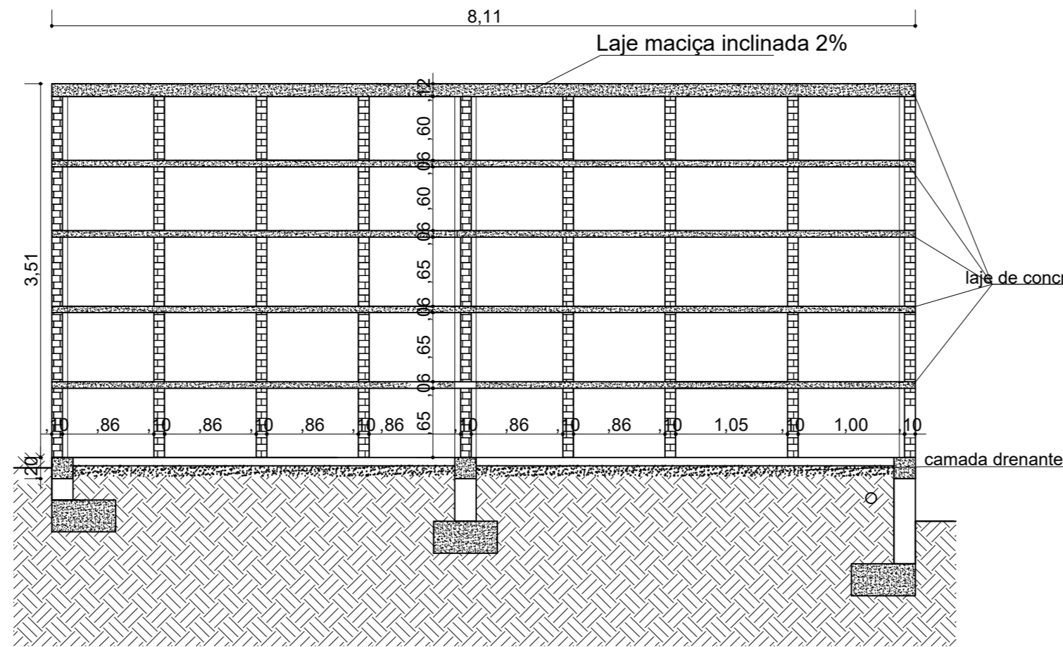
CORTE LONGITUDINAL - BLOCO "A" ESC.: 1/50
