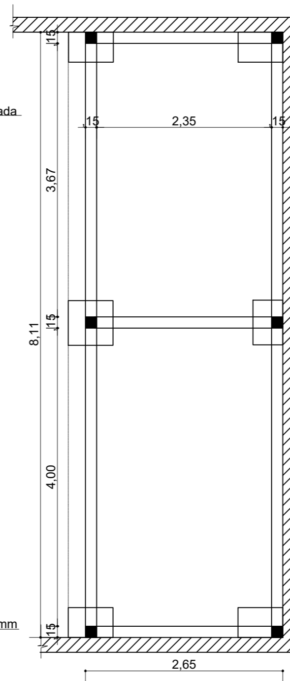
PLANTA DE FORMAS BLOCO "A" ESC.: 1/50
