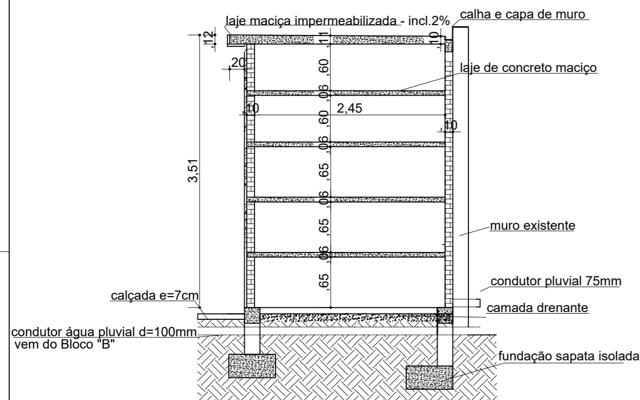
CORTE LONGITUDINAL BLOCO "B" ESC.: 1/50
